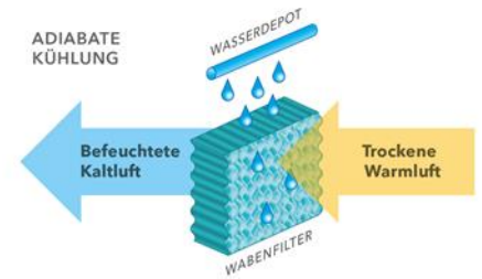
Luftkühler Funktionsprinzip
